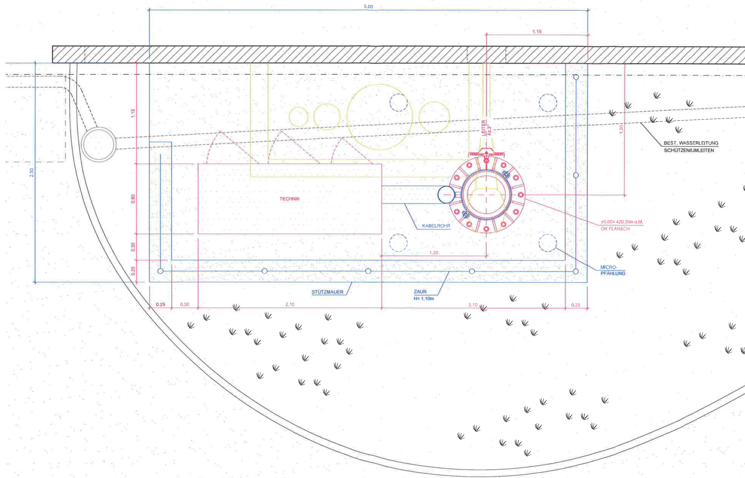
SITUATION 1:25
